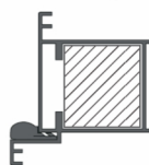
Коробка АЛЮМИНИЙ с заполнением МДФ скрытая
